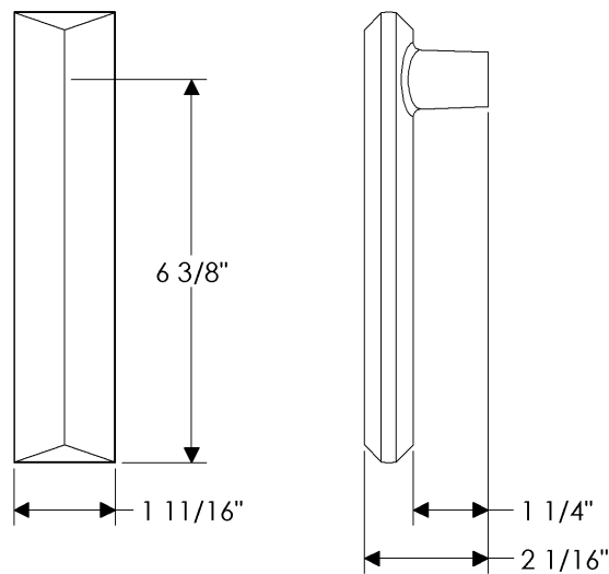
L21075 Long Emile Lever
